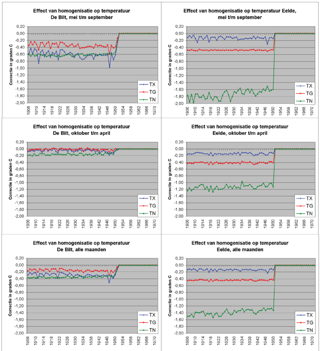
Figuur 2. Effect van homogenisatie op de temperatuurreeksen van De Bilt en Eelde voor de zomermaanden, wintermaanden en het gehele jaar. De verticale as geeft de gemiddelde correctie per jaar van de dagelijkse maximum temperatuur (TX), dagelijkse gemiddelde temperatuur (TG) en dagelijkse minimum temperatuur (TN)
