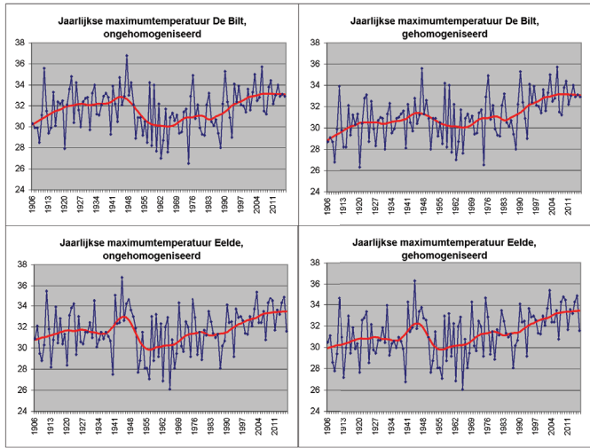
Figuur 3. Effect van homogenisatie op de jaarlijkse maximumtemperatuur (TXX) te De Bilt en Eelde. De rode lijn geeft de trendlijn volgens een loess smoothing op basis van een lokaal gewogen regressie over 20 punten.
