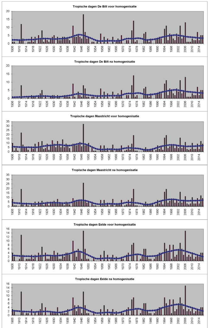
Figuur 4. Het aantal tropische dagen per jaar (TX ≥ 30 °C) voor De Bilt, Maastricht en Eelde, voor en na de homogenisatie. De vloeiende lijnen geven de trend volgens een loess smoothing op basis van een lokaal gewogen regressie over 20 punten.
