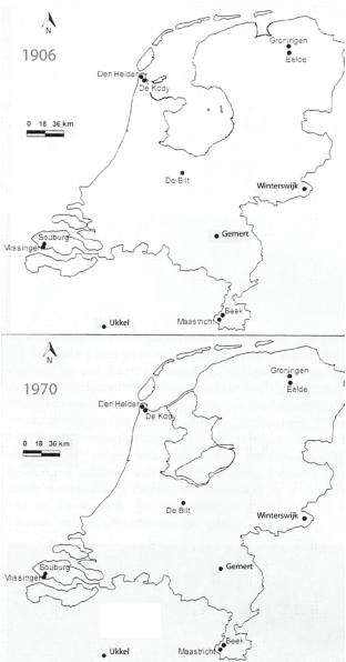
Figuur 1. Locatie van de 5 hoofdstations ten opzichte van Zuiderzee/IJsselmeer en Lauwerszee in 1906 respectievelijk 1970. Bewerkt naar Brandsma (2016a). Toegevoegd zijn de in het artikel genoemde stations Gemert, Winterswijk en Ussel (België).
